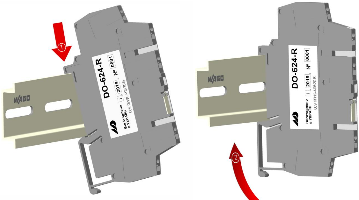
Рисунок 3.2 – Схема крепления модуля DO-624-R на DIN-рейке
