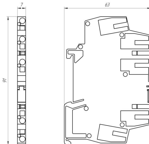
Рисунок 1.1 – Внешний вид и габаритные размеры модуля DO-624-R
