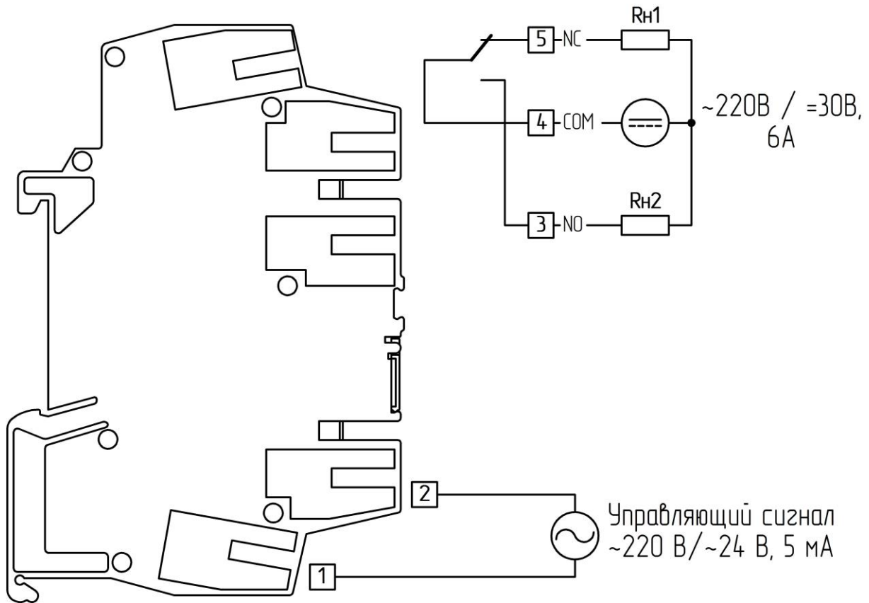
Рисунок 3.4 - Схема внешних соединений модуля DO-624-R
