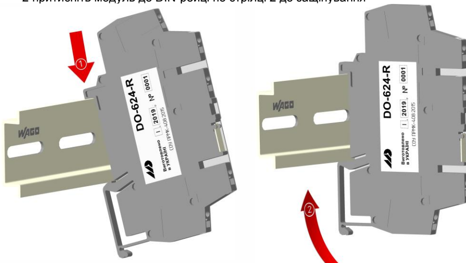
Рисунок 3.2 - Схема кріплення модуля DO-624-R на DIN-рейку
