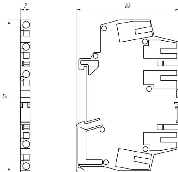
Рисунок 1.1 - Зовнішній вигляд і габаритні розміри модуля DO-624-R
