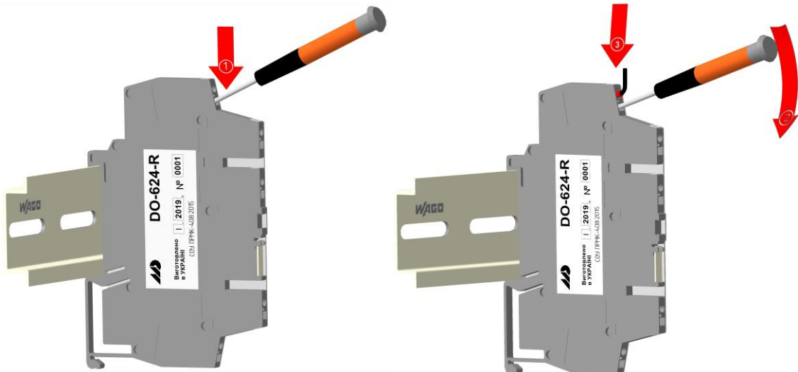
Рисунок 3.3 – Підключення проводів за допомогою плоскої викрутки
