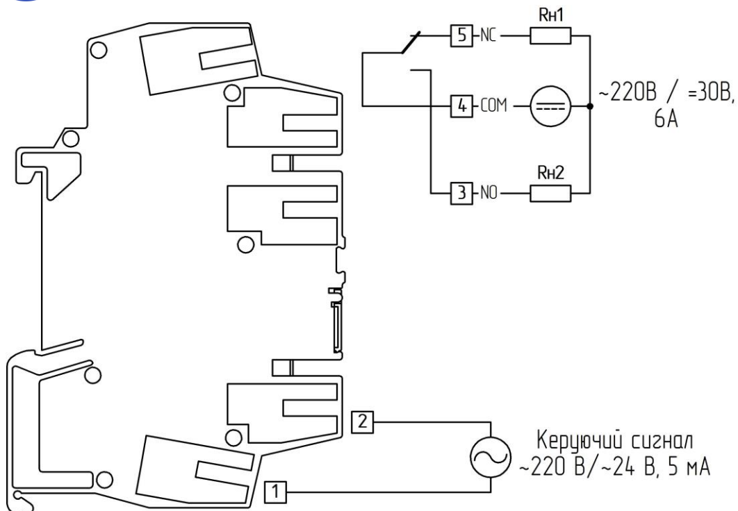
Рисунок 3.4 - Схема зовнішніх з'єднань модуля DO-624-R
